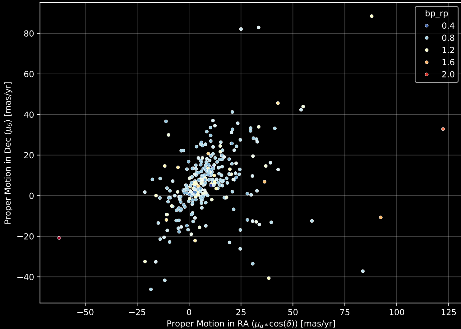
GALAH DR4 Field: [205] Proper Motion Diagram (n= 302)
