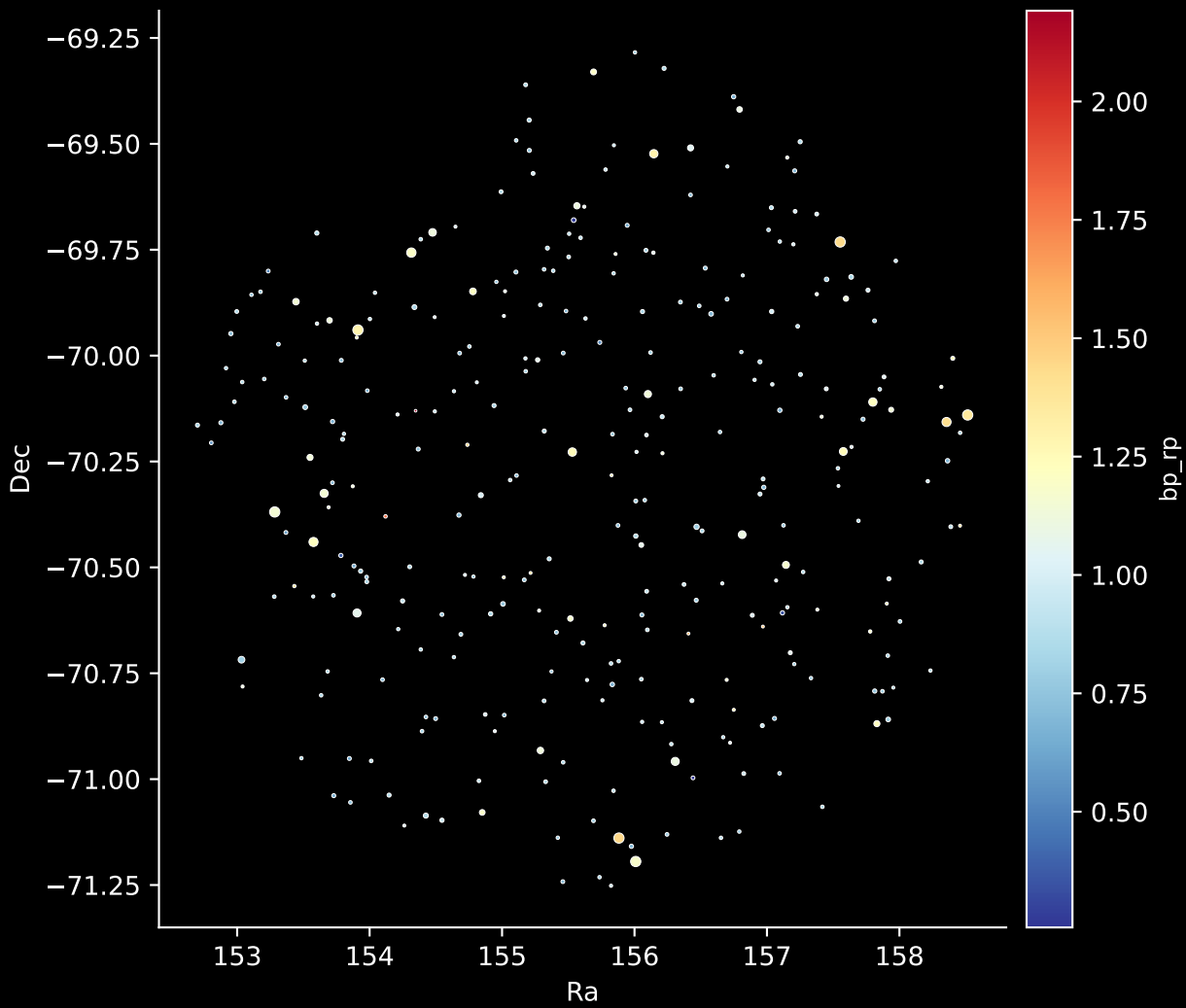
GALAH DR4 Field: [205] Stars: 302
