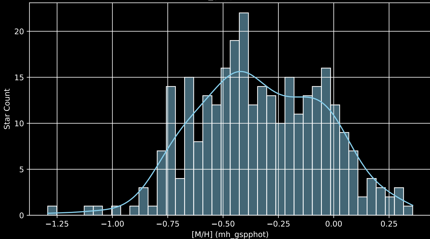
GALAH DR4 Field: [205] [M/H] (mh_gspphot) (n= 300)
