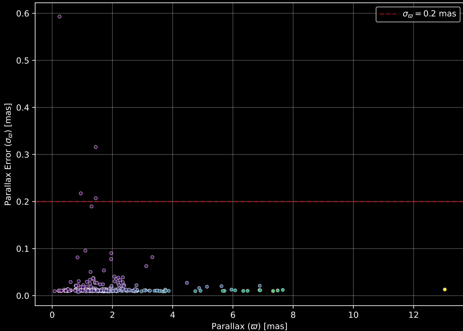
GALAH DR4 Field: [205] Parallax Quality (n= 302)
