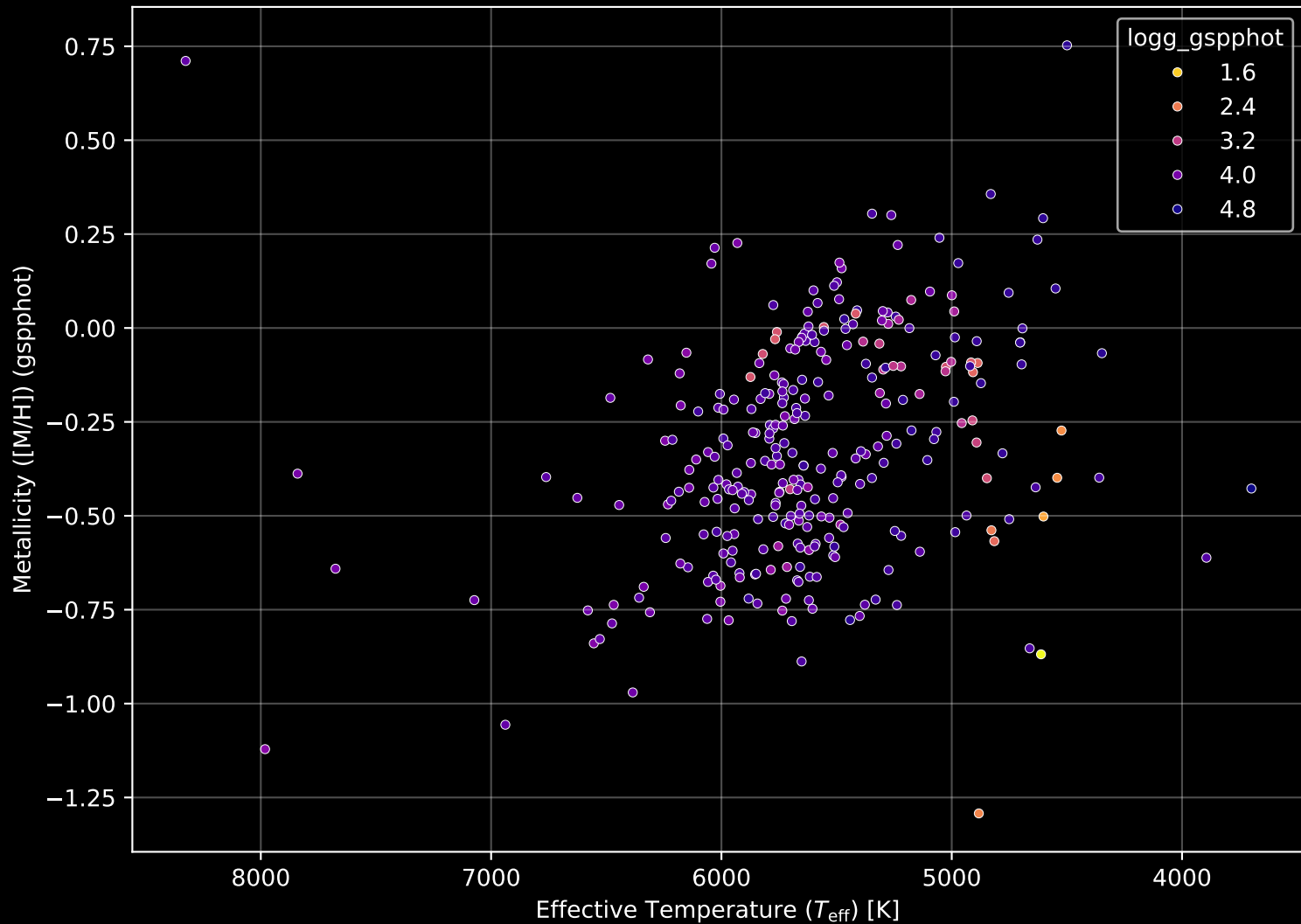
GALAH DR4 Field: [205] Stellar Population Parameters (n= 302)
